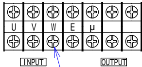
端子配列
